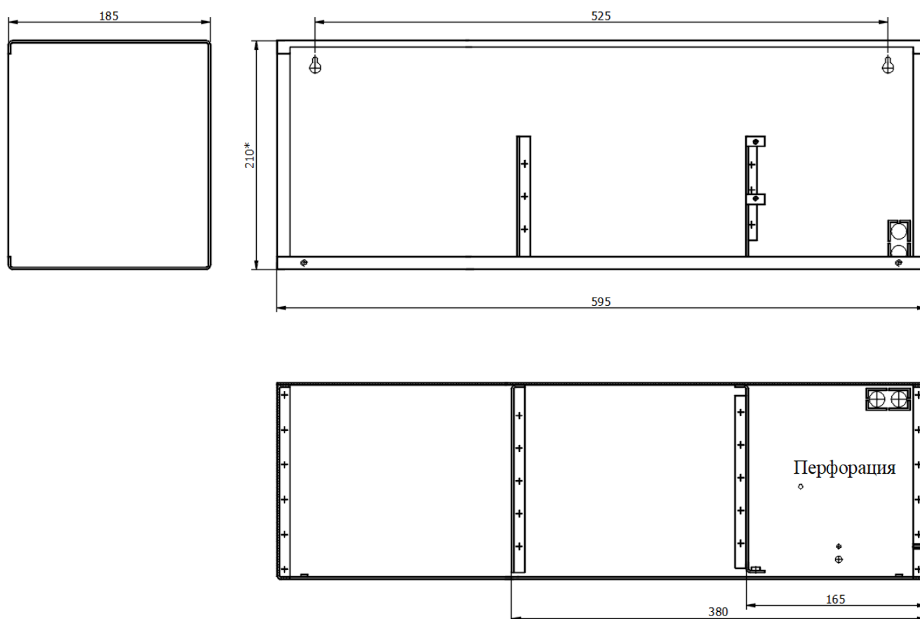
Рисунок 2 - Габаритный чертеж корпуса ТИП-4
